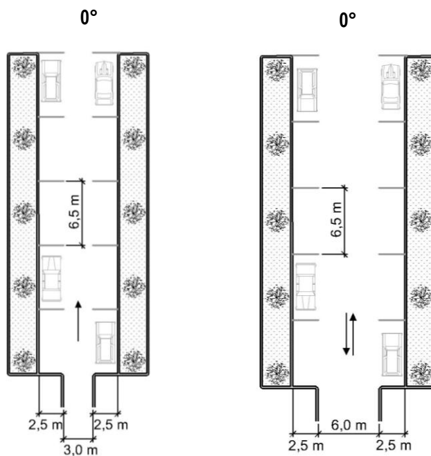
Figure 7-8 - Dimensions relatives aux cases de stationnement, aux allées d'accès et aux allées de circulation
